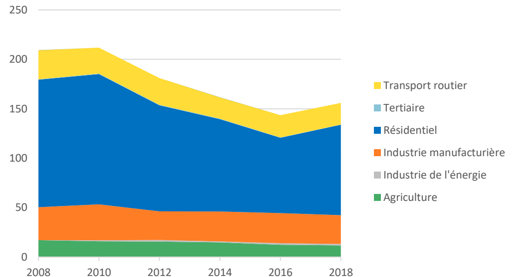
Evolution des émissions de PM2.5 par secteur - Terre d'Emeraude
