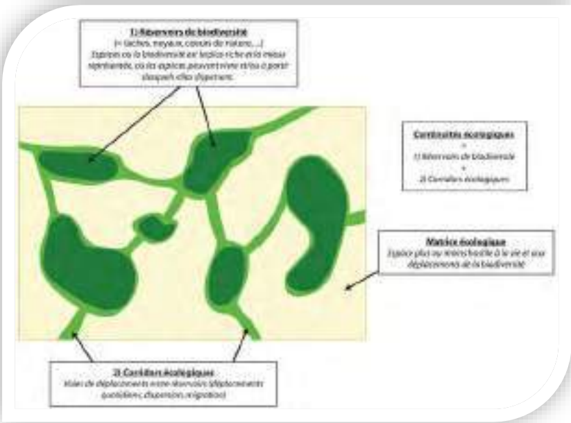
Schéma théorique expliquant les liens entre corridors et réservoirs formant les continuités écologiques –M5-FaunaNat
