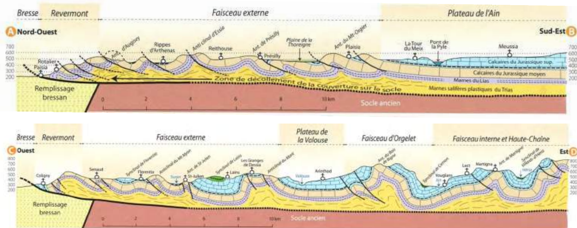
Coupes géologiques de la Petite Montagne du Jura Source : Montagnes du Jura géologie et paysages, Michel Comby & Vincent Brichet, 2008
