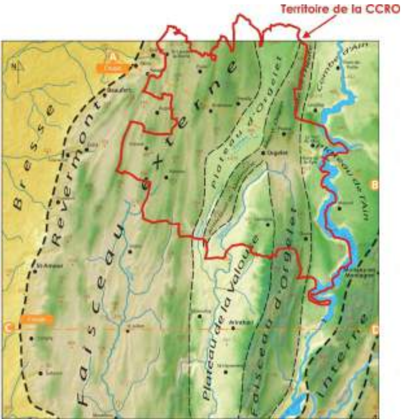
Schéma structural de la région de la Petite Montagne du Jura – Source : Montagnes du Jura, géologie et paysages, Michel Compy & Vincent Pichet, 2008
